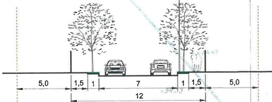
Profil Str. Libelulei conform PUZ Zona de Nord - Sc. 1/200
